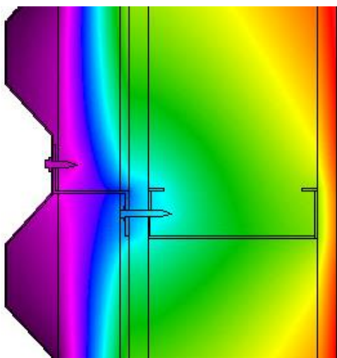
Metal girt
